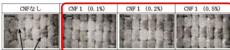
図3 スレ発生の様子(顕微鏡150倍画像)
