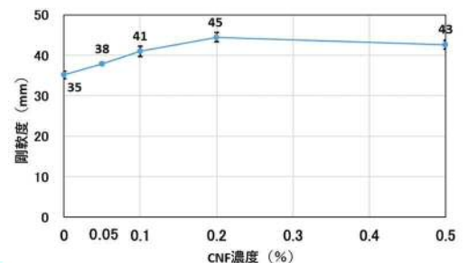
図4 剛軟度試験結果
